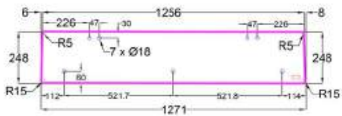
100AS014 AUSA BD 202 LUNETA TRASERA INFERIOR
