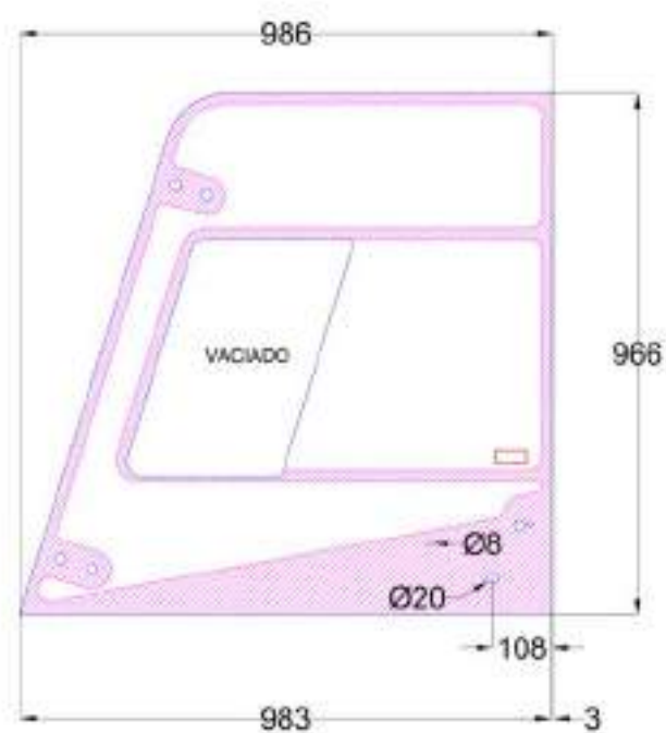
100GT003I ESAGONO GASTONE PUERTA IZQUIERDA
